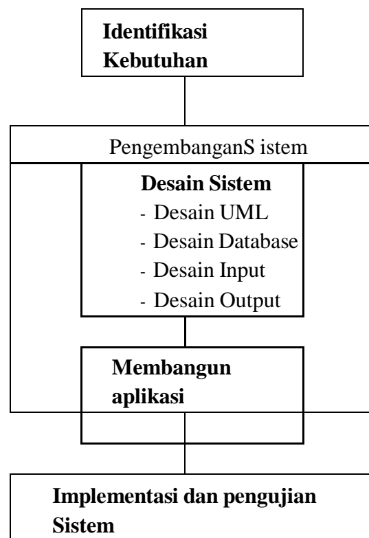
Gambar 2. Metodologi penelitian
