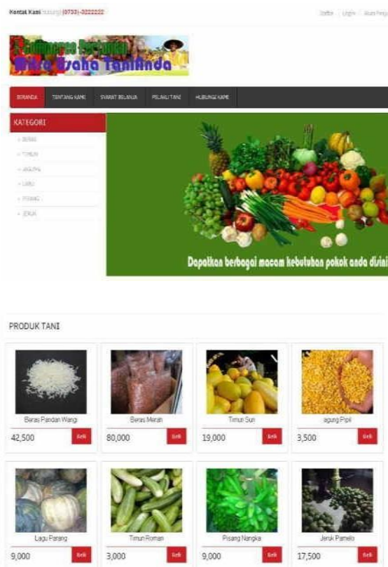
Gambar 5. Halaman Utama
