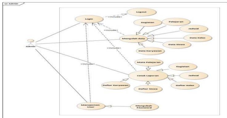
Gambar 2.3 Use case pada diagram Admin
