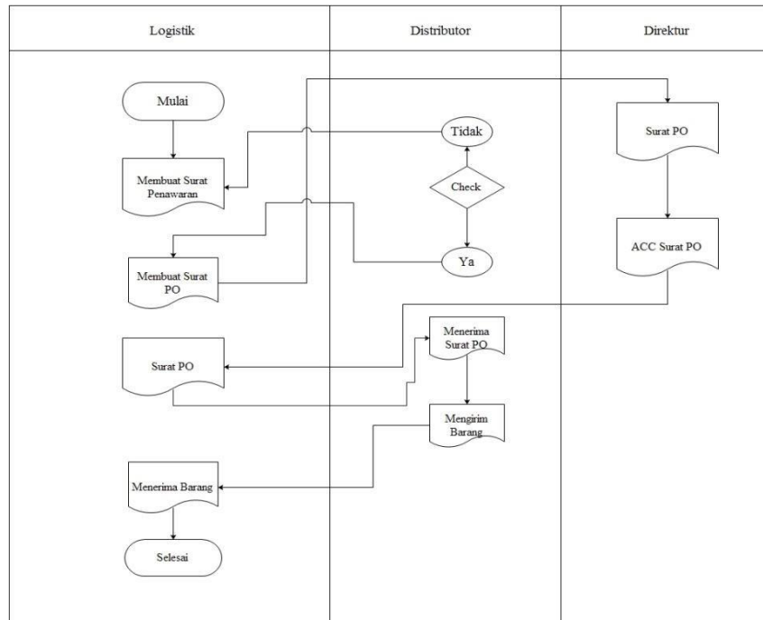
Gambar 4.1 Sistem Pembelian dan Penjualan yang sedang berjalan
