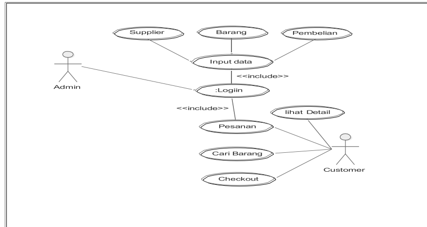
Gambar 3.3 Use Case Diagram Pembelian dan Penjualan Sparepart
